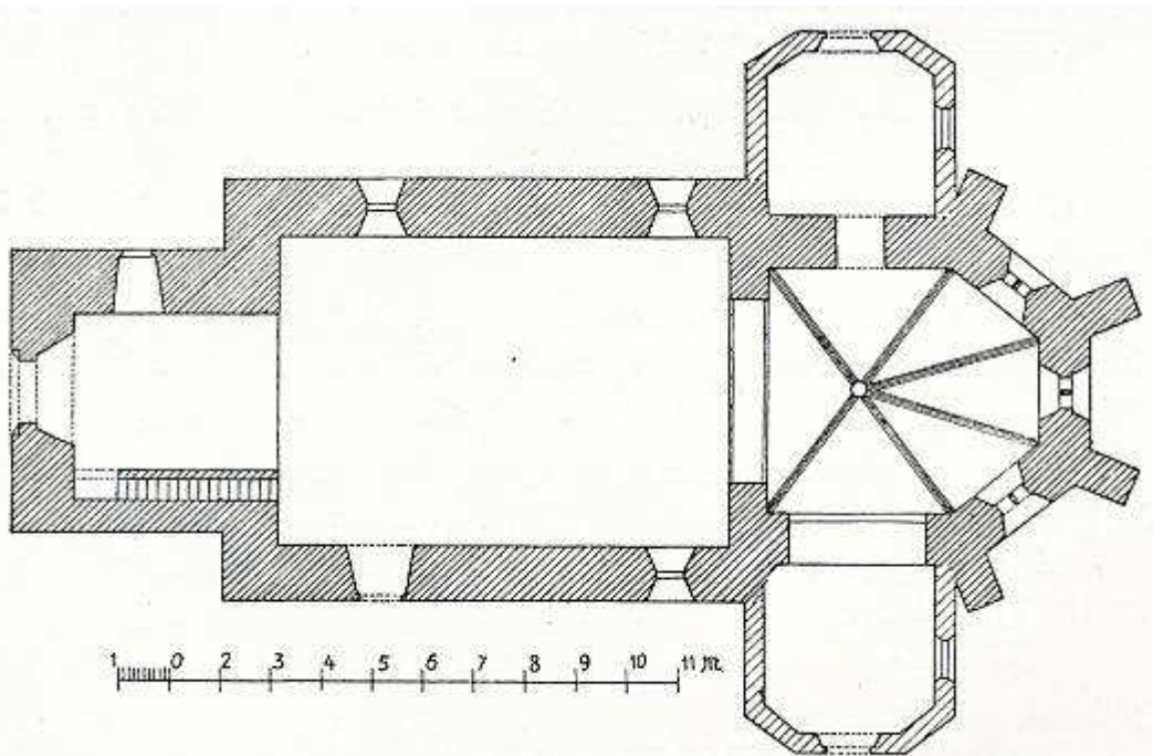
Obr. 86 Ratměřice. Půdorys kostela.
